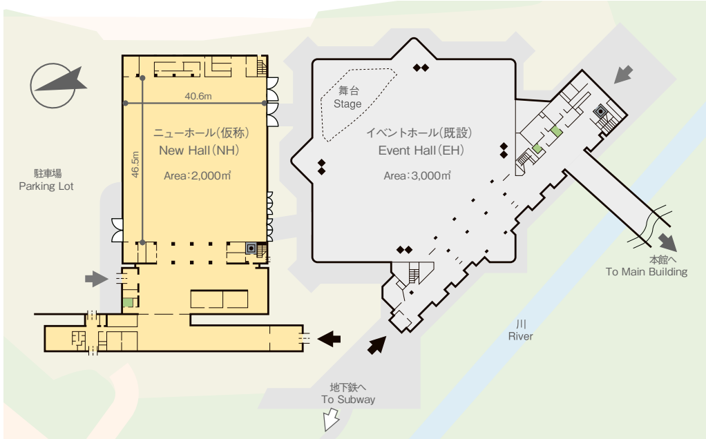
平面図 Floor Plan
